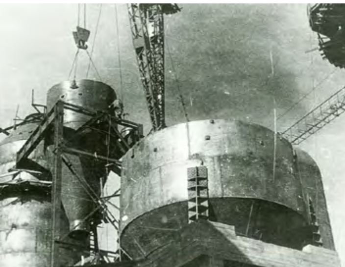
Строительство комплекса комсомольской доменной печи №6 на Магнитогорском металлургическом комбинате в 1943 году. Установка нижней части циклона.
